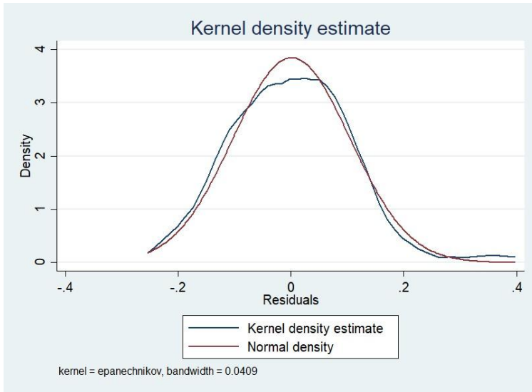
ღანართი 4. Kernel density estimate
