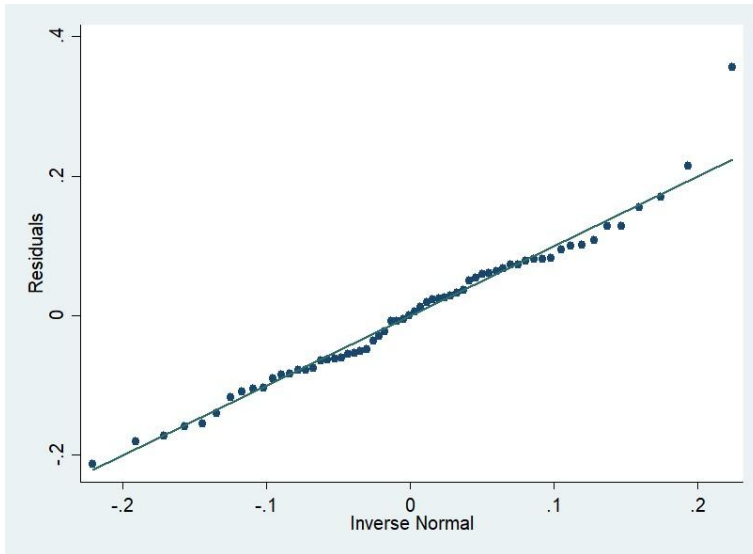
ღანართი 5. pnorm r2012
